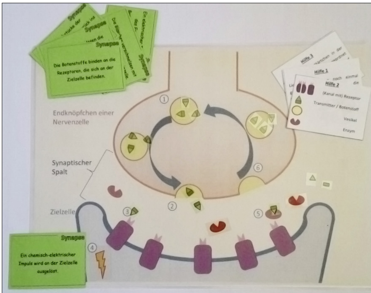
Abb. 14: Synapsenspiel
